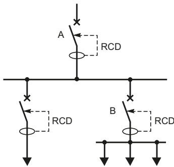
Fig. F15 Distribution circuits
