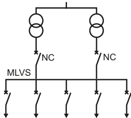
Fig. D21 Parallel transformers configuration
