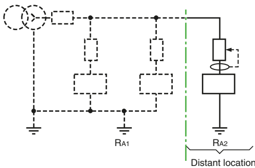
Fig. F16 Separate earth electrode
